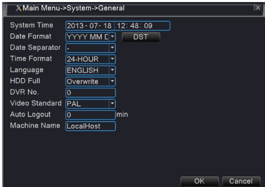
Рис. 4.13 Общие настройки
