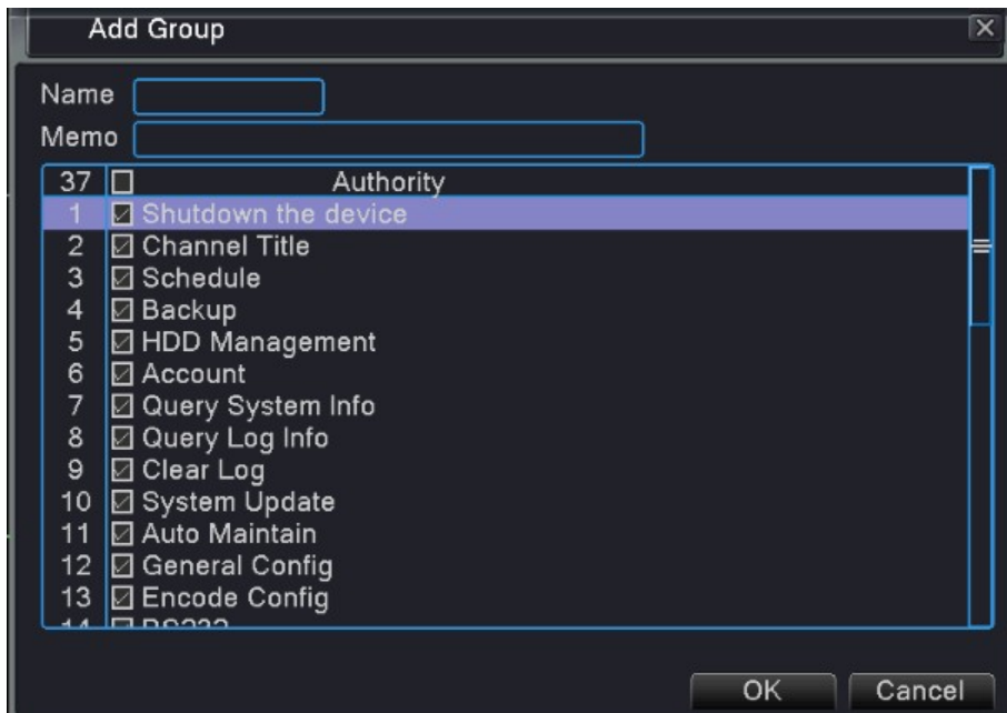
Рис.4.49 Добавление группы
