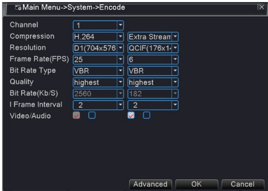
Рис. 4.14 Настройка кодировки
