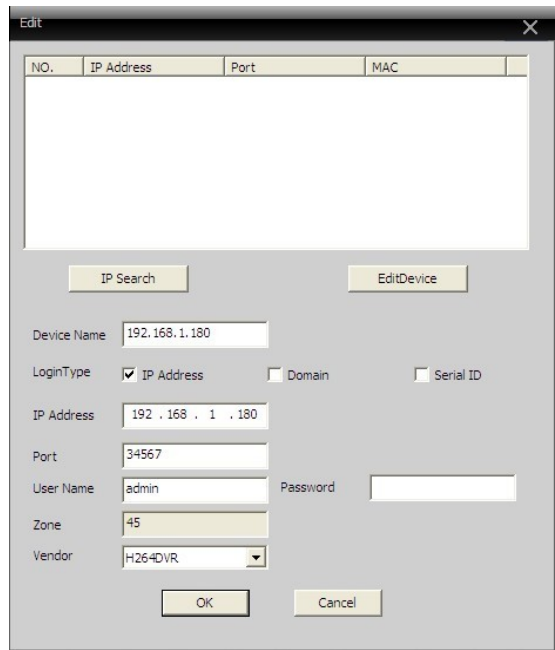
Рис. 5.10 Редактирование
